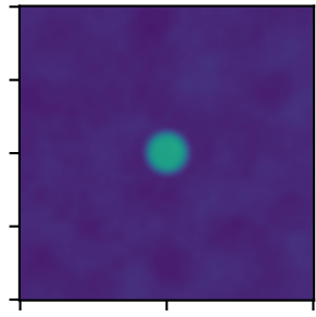
TrapezoidDisk2DKernel
