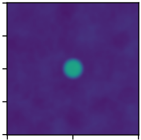
TrapezoidDisk2DKernel
